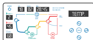
CONTROLADOR ELECTRÓNICO PROGRAMABLE ARMARIO FERMENTACIÓN CONTROLADA
