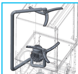
Bomba de doble flujo
