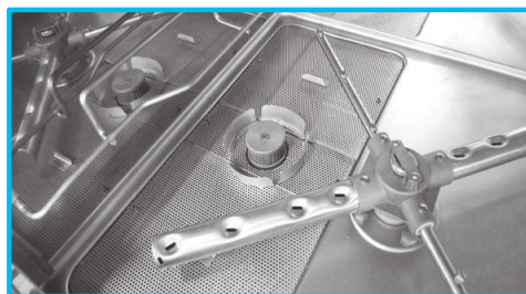
Prefiltros desmontables (solo PM-50)
