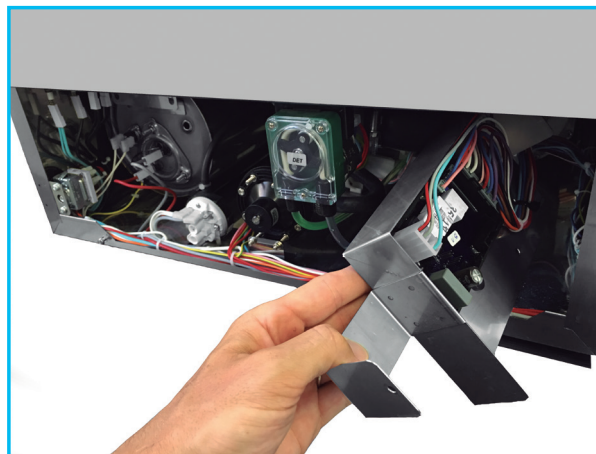
Componentes en la zona inferior frontal de la máquina para facilitar el acceso.
